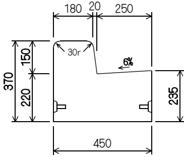
切り下げ型
