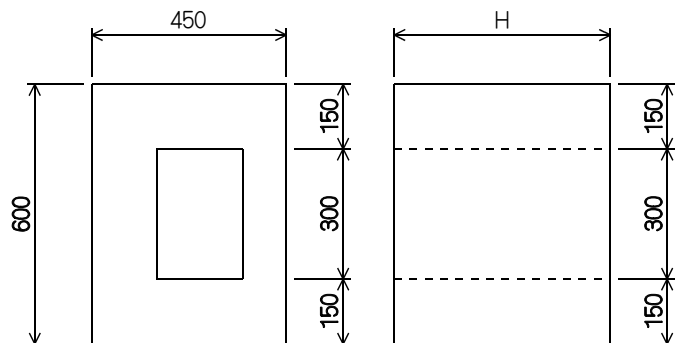
下部柵
