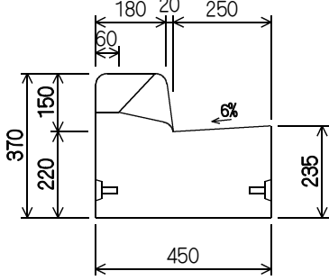
すり付け型
