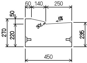
すり付け型
