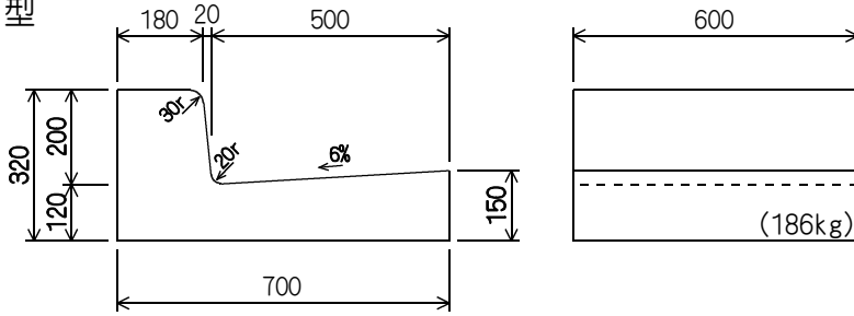
MD-B1
