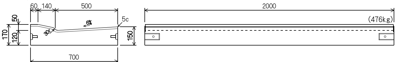
MD-B1(L=2000)
