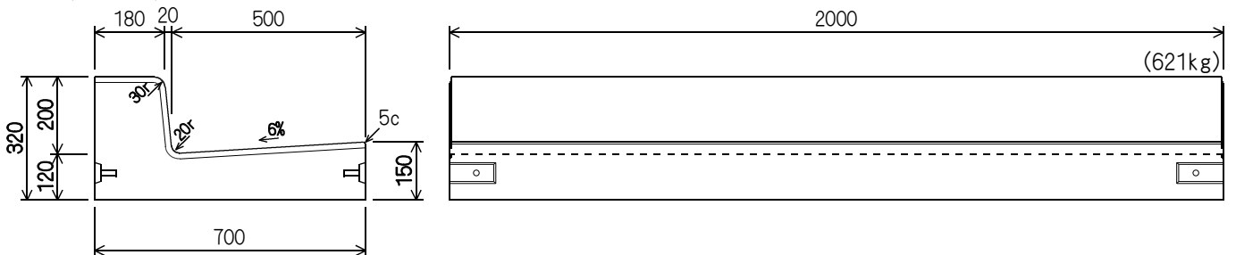
MD-B1(L=2000)
