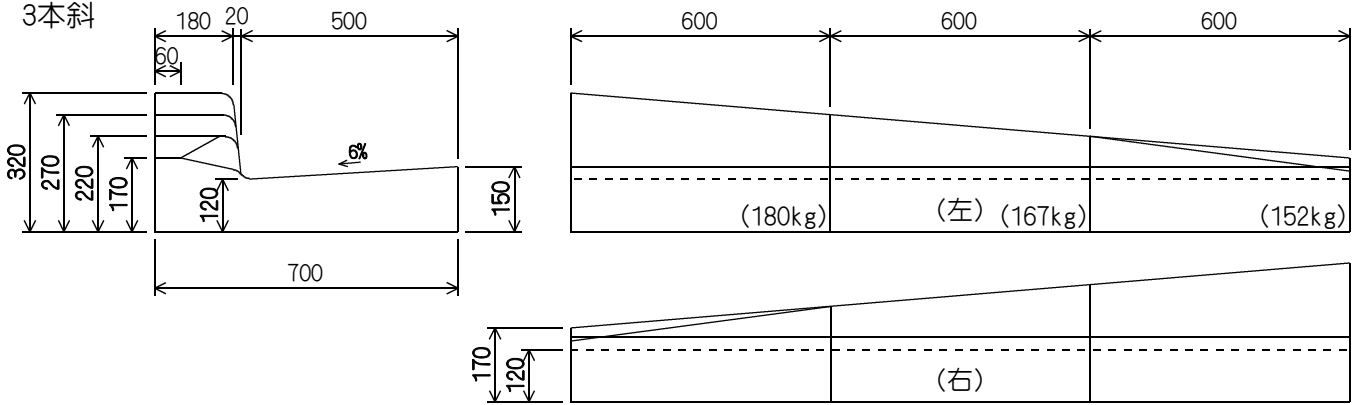
II型(L=2000)
