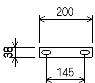
連結プレート
