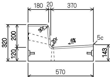
一般型 (L=2000) 水抜き付
