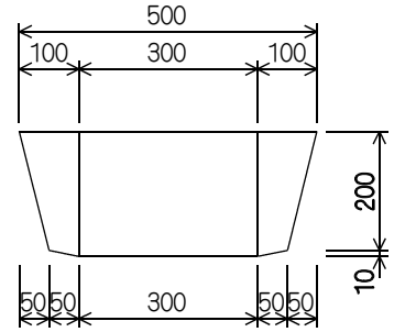
側塊(異形)
