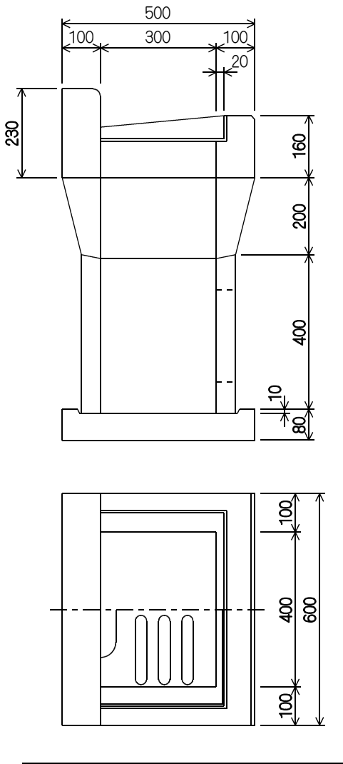
組立図
