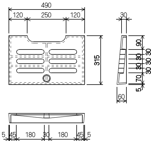
ふた(鑄鉄)
