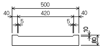
底塊
