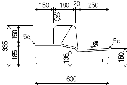
SFT-B1タイプ (斜)
