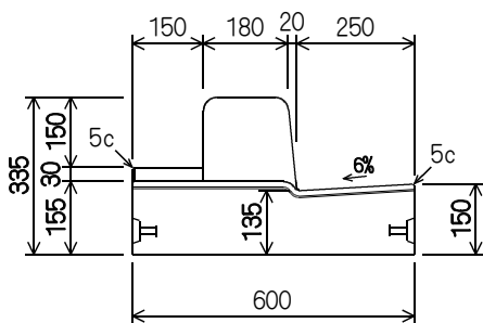
SFT-BH20タイプ (斜)
