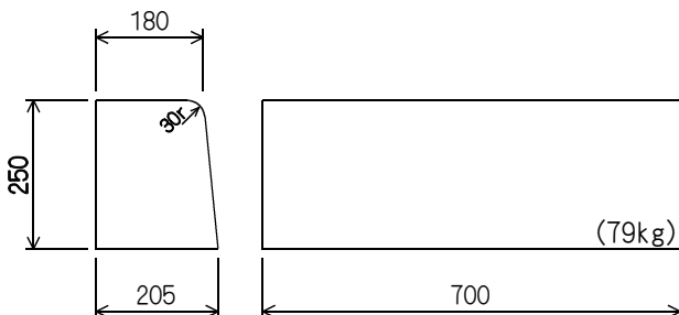
片面歩車道境界ブロック B (L=700)
